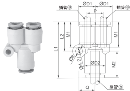
C-KQ2U U型接管
