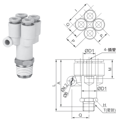
C-KQ2UD 外螺Y型五通接头
