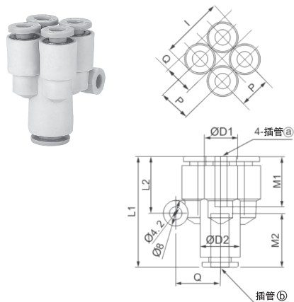
C-KQ2UD变径五通接管
